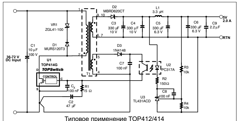
Типовое применение TOP412/414
